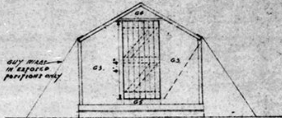
END ELEVATION
